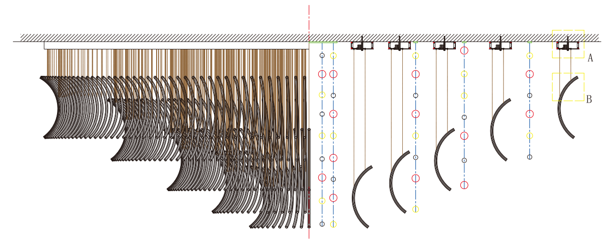
正视图 front view
